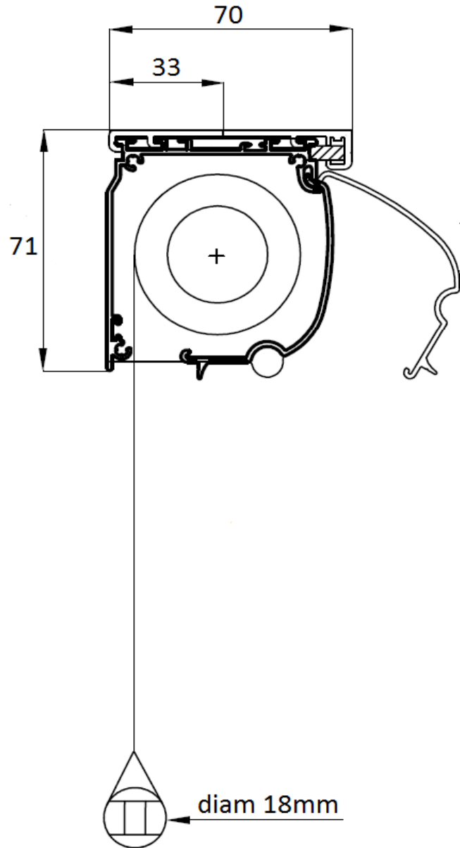
Sunbox 63 - Vue de coupe pose plafond:
