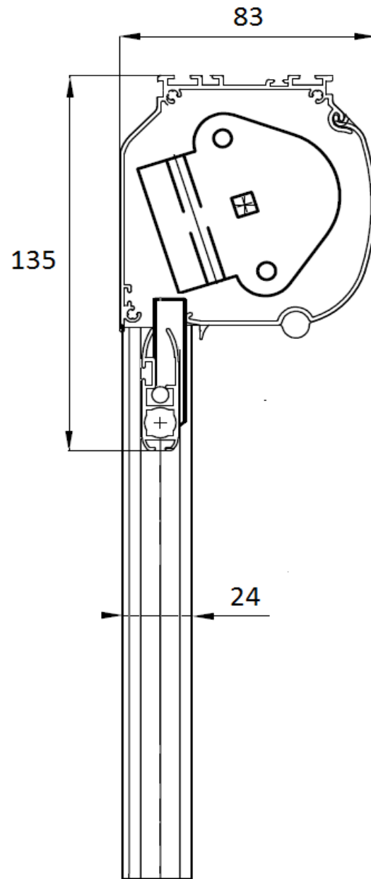
Sunbox 83 - Vue de Coupe store enroulé:
