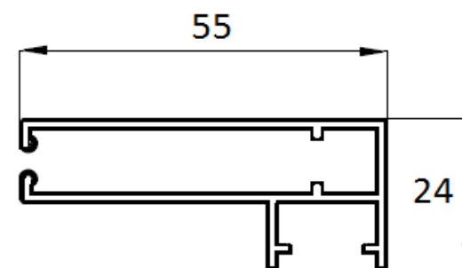
Détail coulisse occultante OC pose de face:
