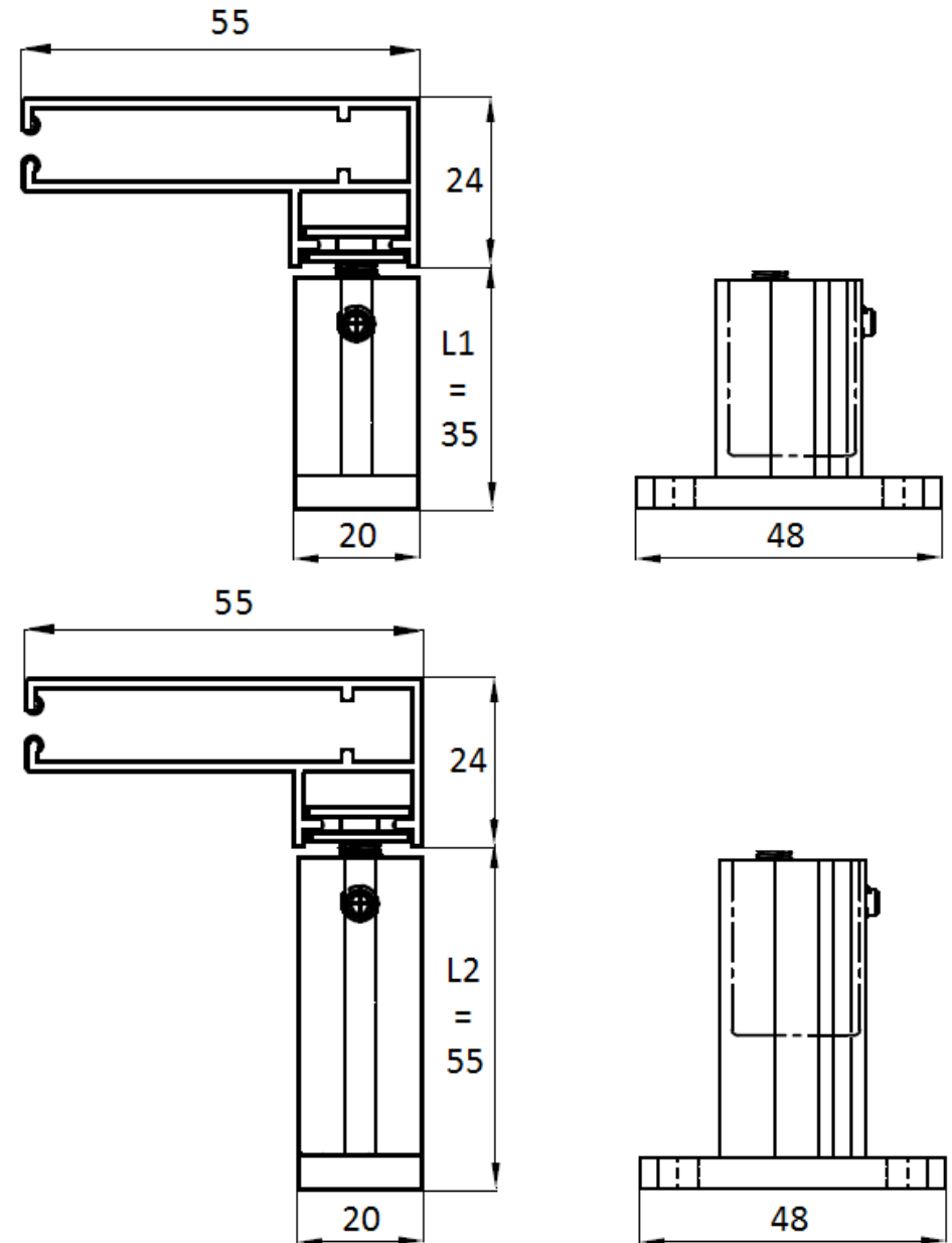
Détail équerre coulisse L1 et L2:
