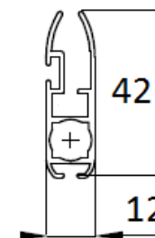
Détail barre de charge plate 42 x 12mm:
