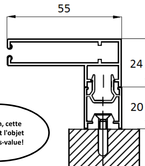
Ensemble profilé déport + coulisse + barre de charge
