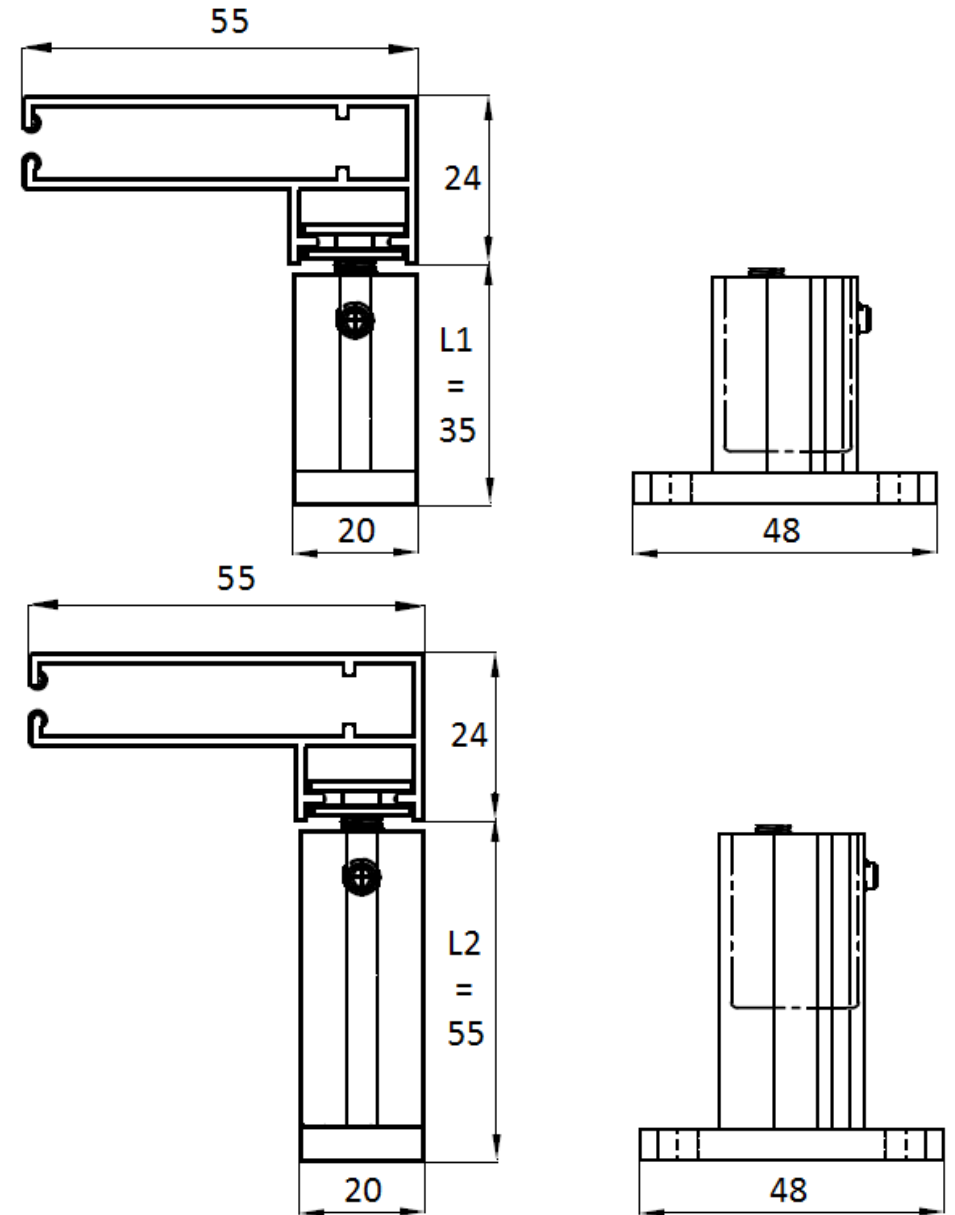
Détail équerre coulisse L1 et L2:
