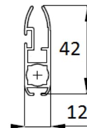
Détail barre de charge plate 42 x 12mm:
