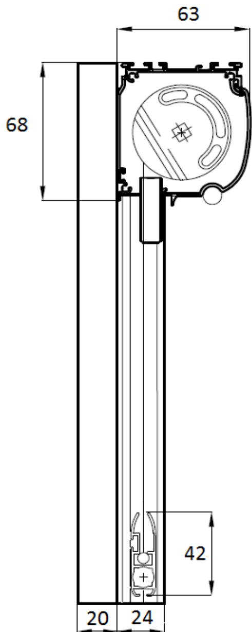
Sunbox 63 - Vue de coupe avec simple profilé:
