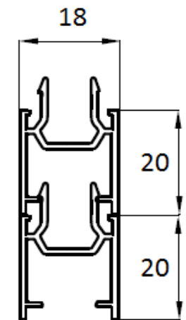
Double profilés:
