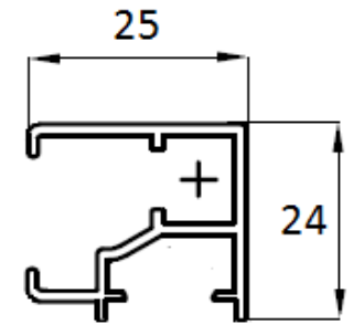
Détail coulisse solaire SO Sunbox 63:
