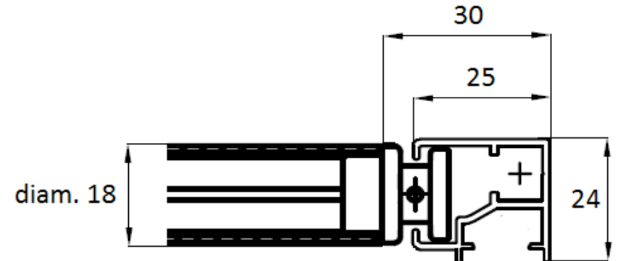
Détail coulisse solaire SO Sunbox 63 + barre de charge:
