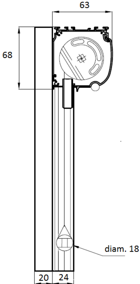
Sunbox 63 - Vue de coupe avec simple profilé:
