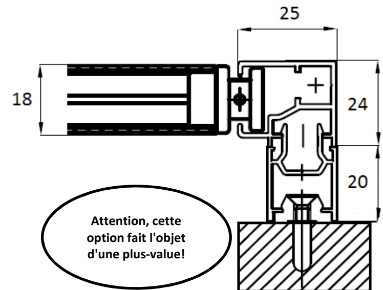
Ensemble profilé déport + coulisse + barre de charge
