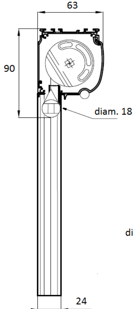
Sunbox 63 - Vue de Coupe store enroulé:
