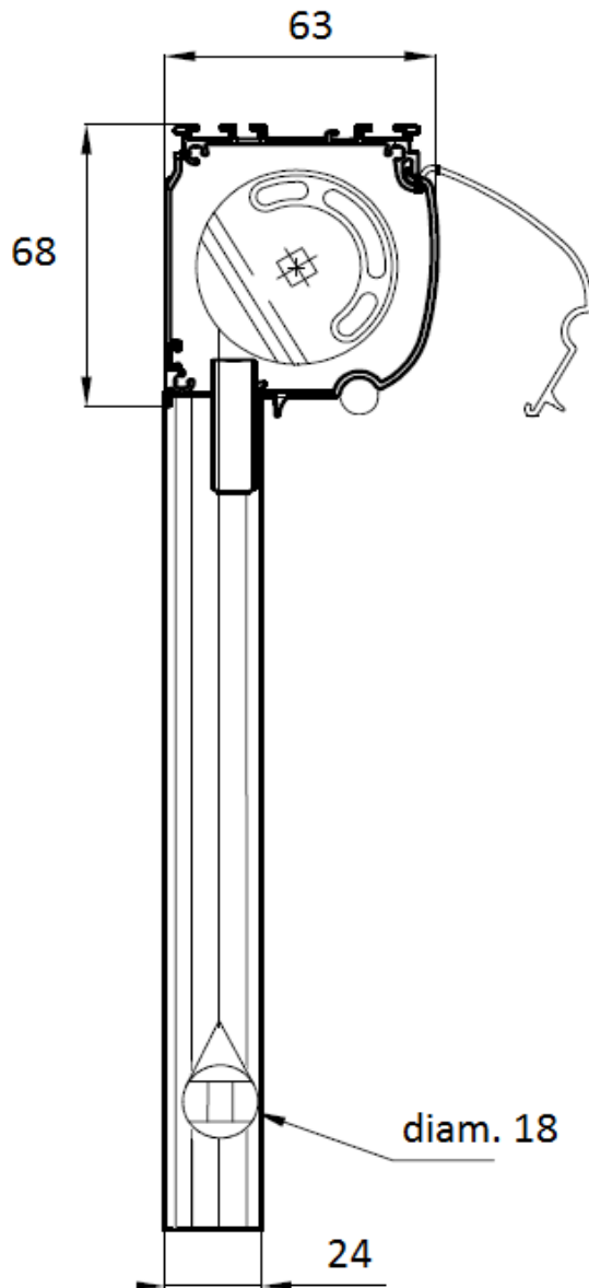
Sunbox 63 - Vue de coupe store déroulé:
