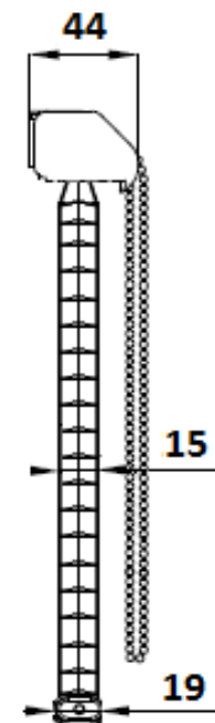
Vue de côté - Pose de face:
