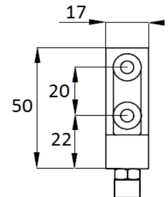
Détail équerre de guidage:
