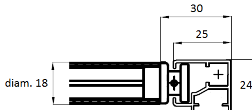
Détail coulisse solaire SO Sunbox 83 + barre de charge:
