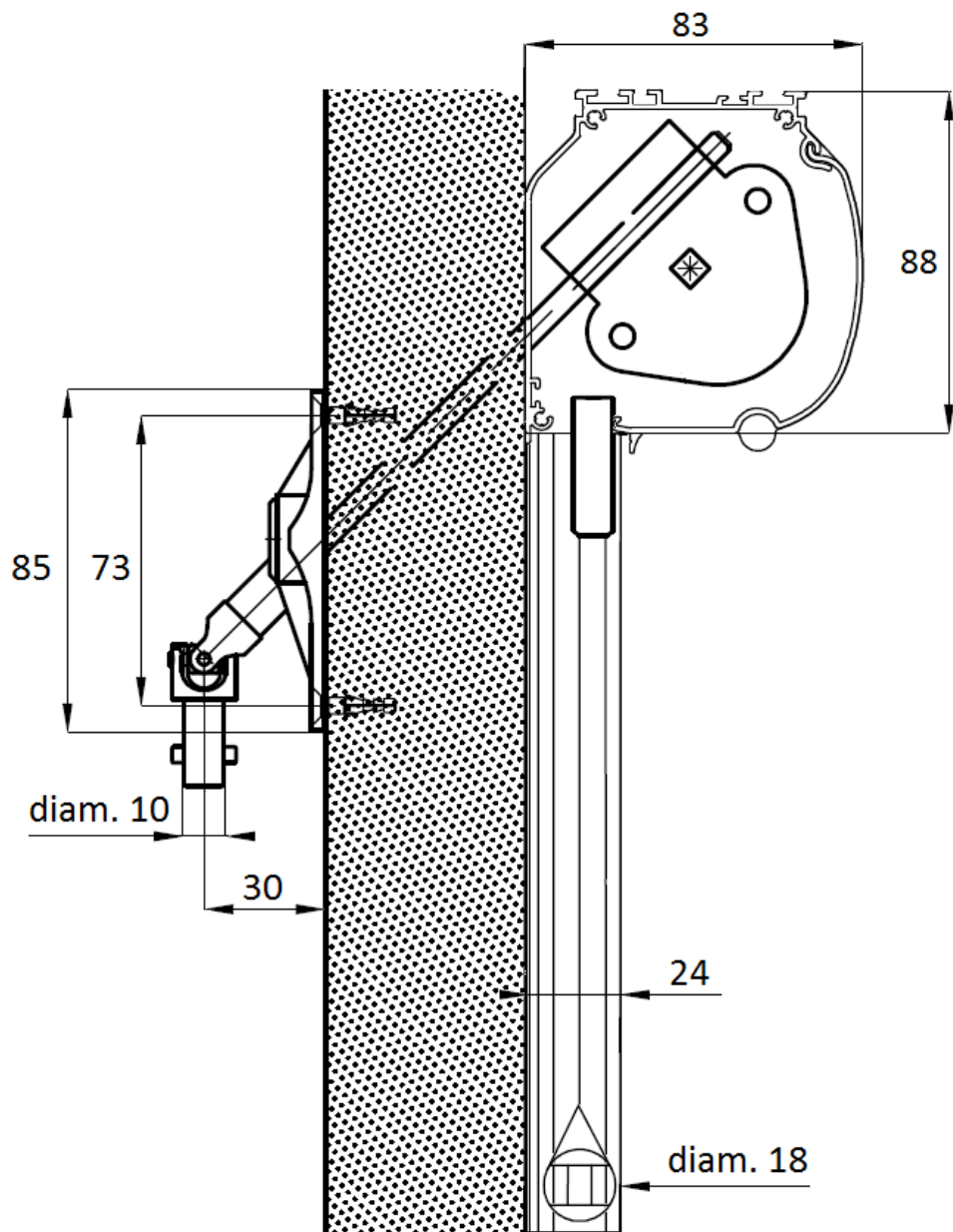
Sunbox 83 avec genouillère renvoi à 45° - Vue de coupe store déroulé:
