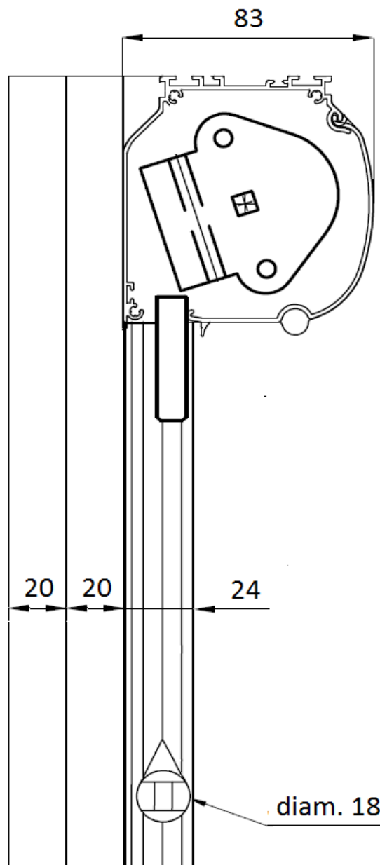
Sunbox 83 - Vue de coupe avec double profilés:
