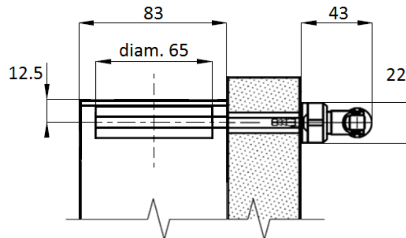
Vue de dessus genouillère avec renvoi intérieur à 90°:
