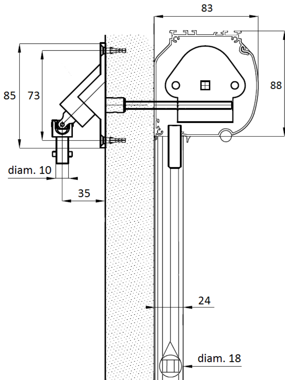
Sunbox 83 avec genouillère renvoi à 90° - Vue de coupe store déroulé:
