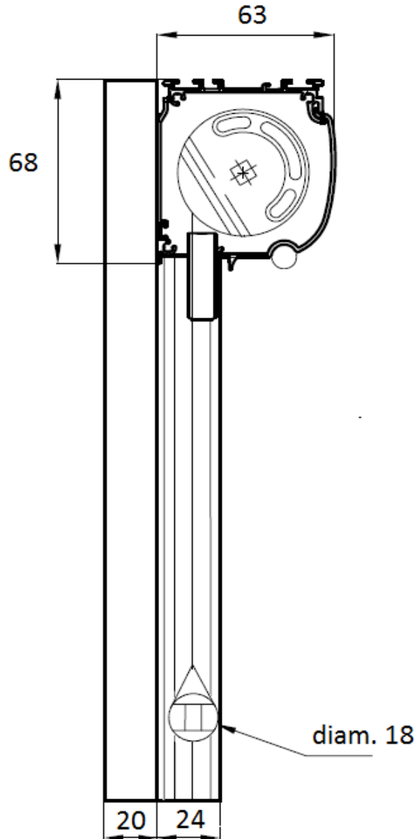
Sunbox 63 - Vue de coupe avec simple profilé:
