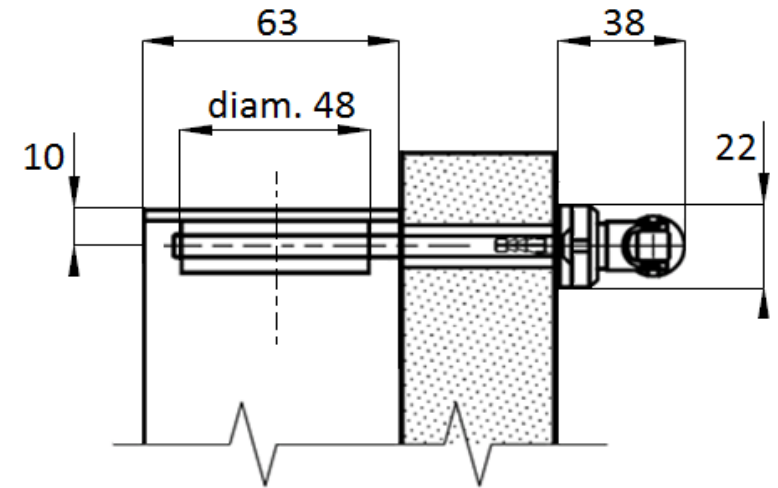
Vue de dessus genouillère avec renvoi intérieur à 45°:
