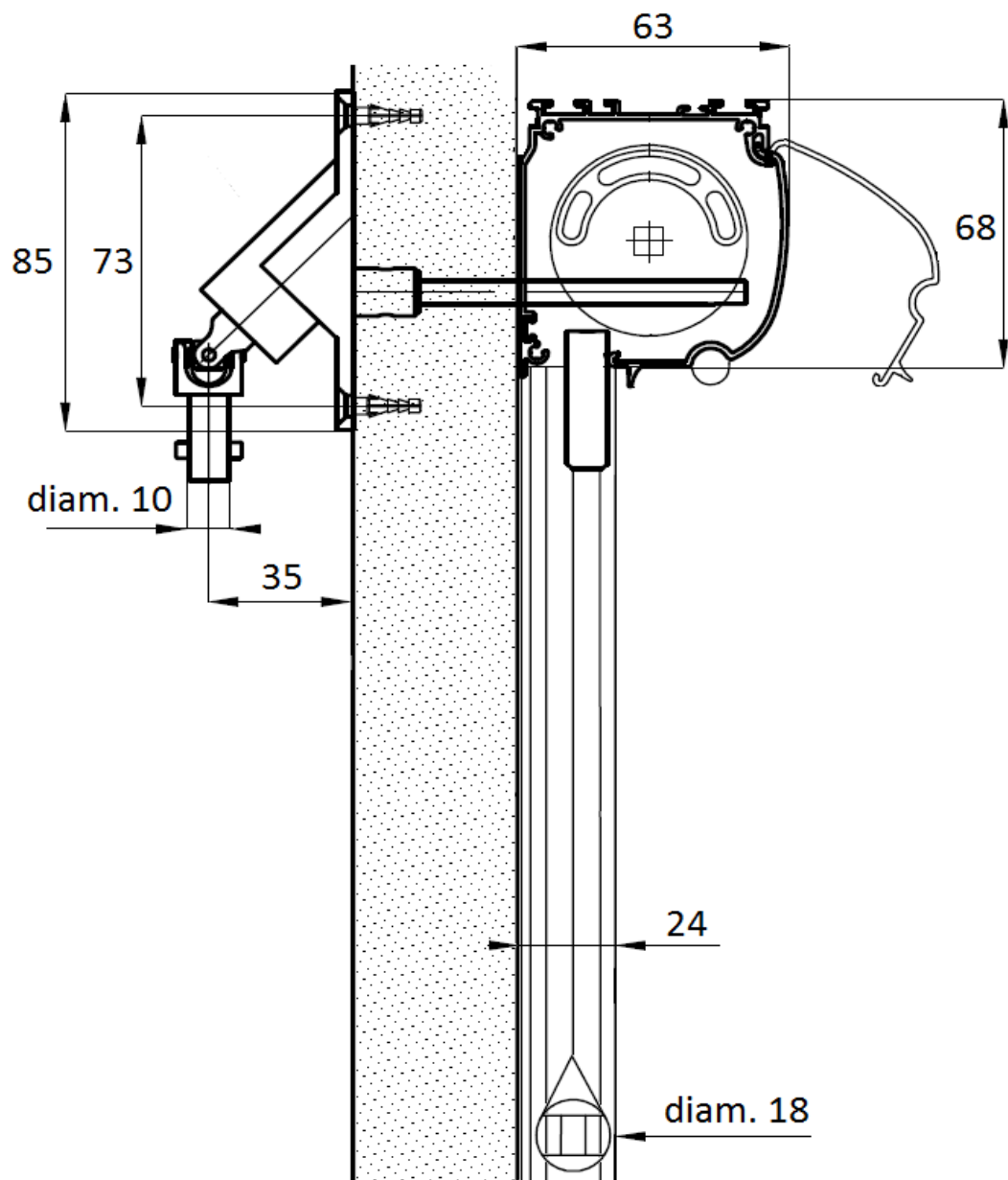
Sunbox 63 avec genouillère renvoi à 90° - Vue de coupe store déroulé:
