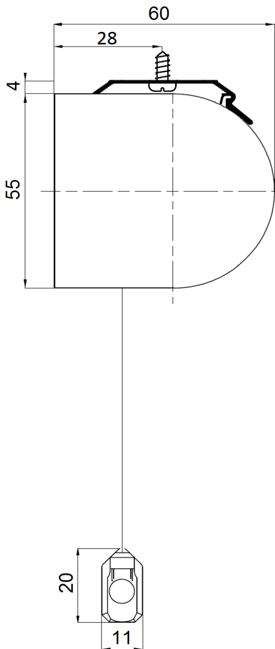
Rouleau Coffre - Vue de coupe pose plafond:
