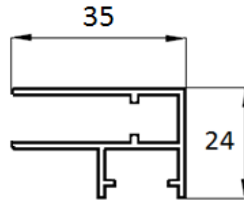
Coulisse solaire SO pose de face:
