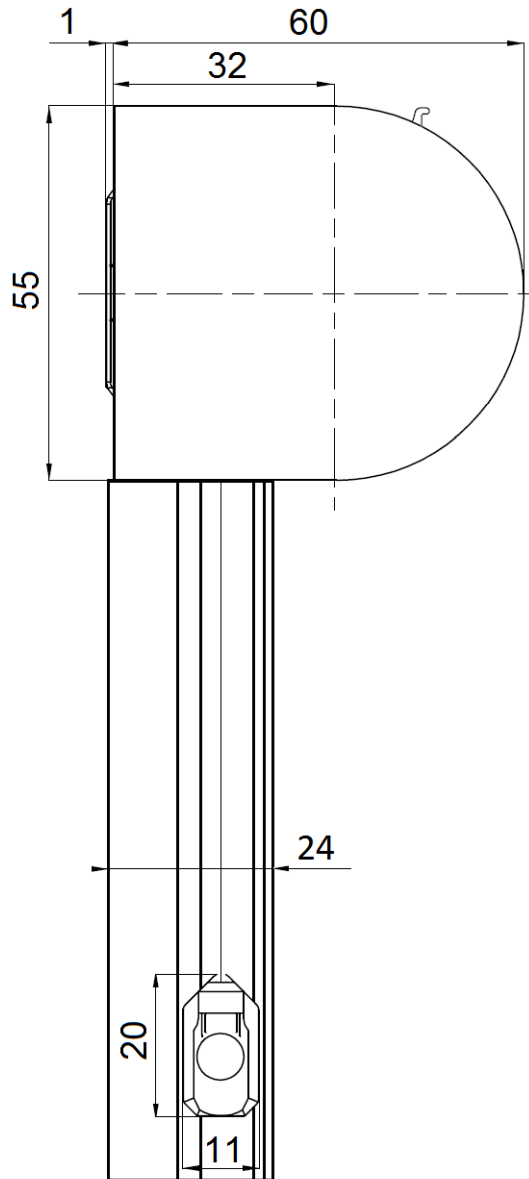
Rouleau Coffre - Vue de coupe pose de face:
