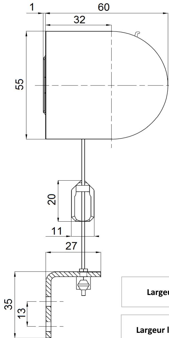
Rouleau Coffre - Vue de coupe pose de face:
