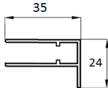
Coulisse solaire SO pose tableau:
