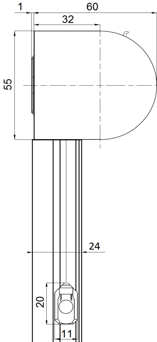
Rouleau Coffre - Vue de coupe pose de face:
