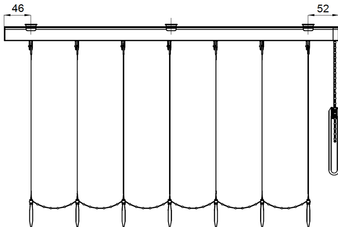
Californien - Vue de face pose plafond:
