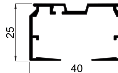
Détail rail supérieur:
