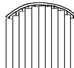
Californien avec rail cintré:
