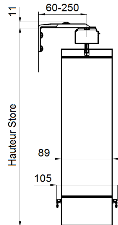
Californien - Vue de côté pose de face:
