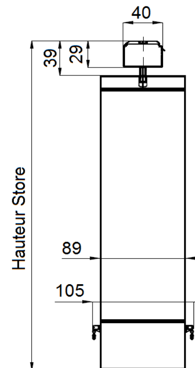
Californien - Vue de côté pose plafond:
