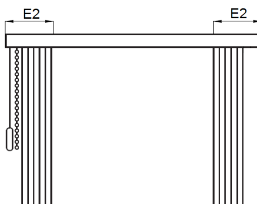
Manœuvre Gauche, Refoulement Côtés:
