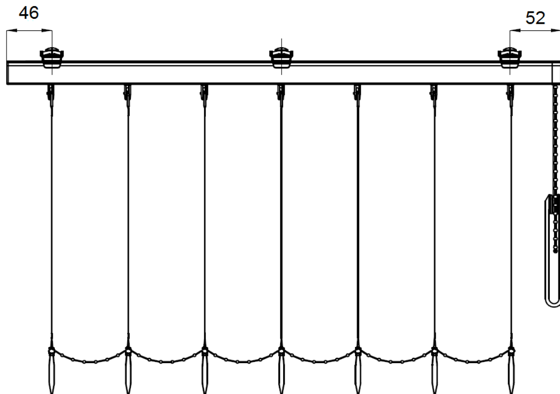
Californien - Vue de face pose de face:
