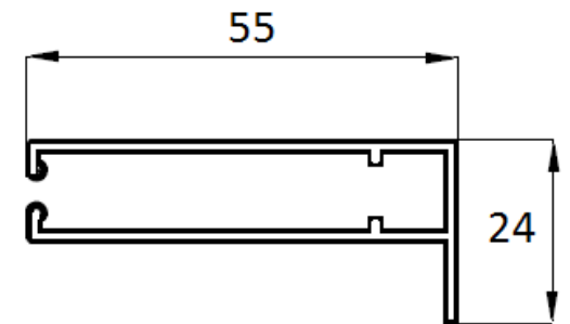
Détail coulisse occultante OC pose tableau:
