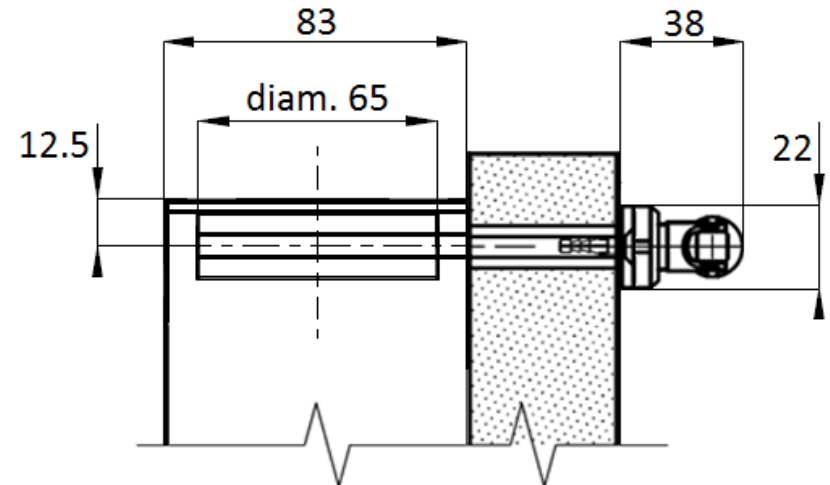
Vue de dessus genouillère avec renvoi intérieur à 45°:
