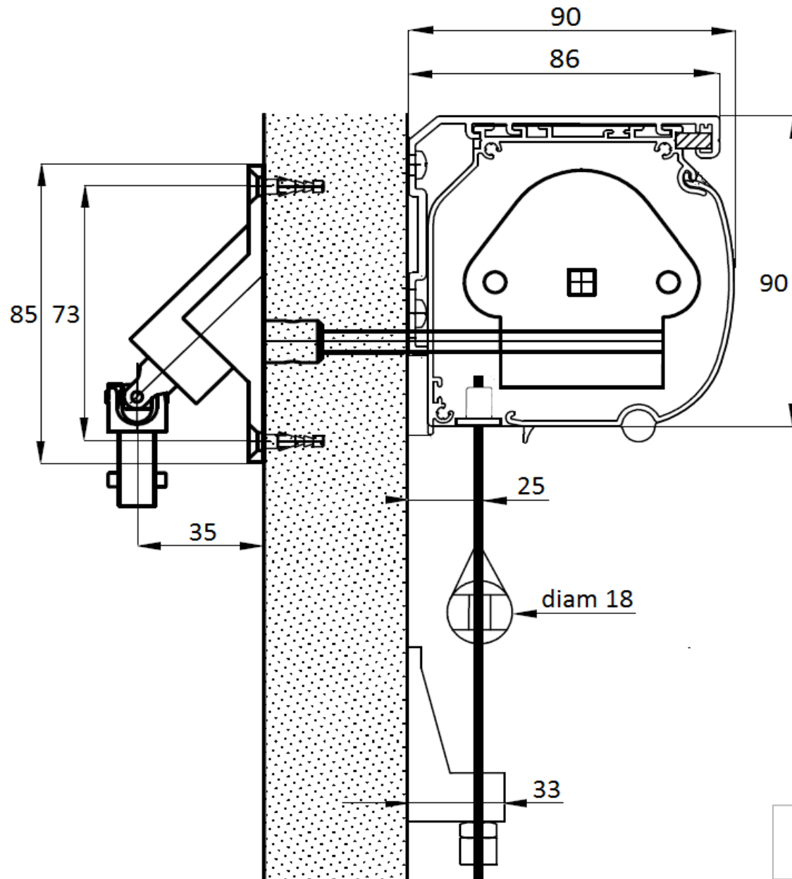
Sunbox 83 avec genouillère renvoi à 90° - Vue de coupe store déroulé:
