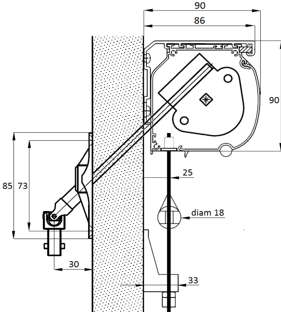
Sunbox 83 avec genouillère renvoi à 45° - Vue de coupe store déroulé:
