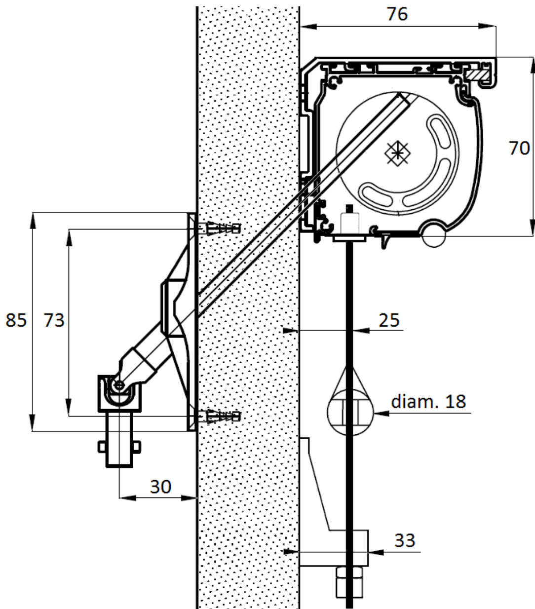
Sunbox 63 avec genouillère renvoi à 45° - Vue de coupe store déroulé:
