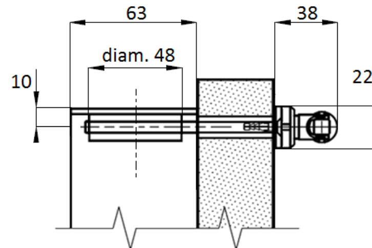
Vue de dessus genouillère avec renvoi intérieur à 45°:
