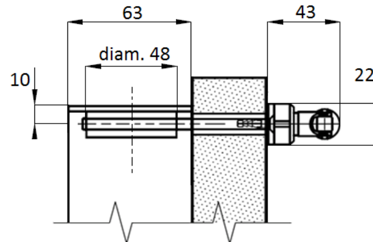
Vue de dessus genouillère avec renvoi intérieur à 90°:
