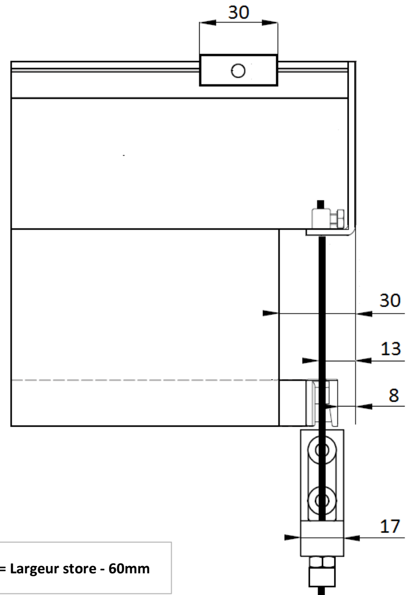
Sunbox 63 avec guidage latéral par câbles- Vue de face:
