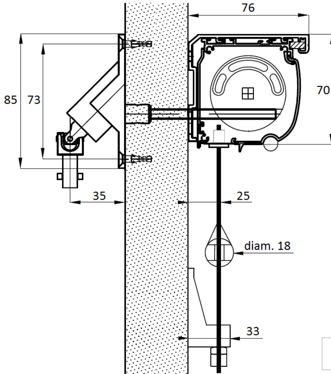
Sunbox 63 avec genouillère renvoi à 90° - Vue de coupe store déroulé:
