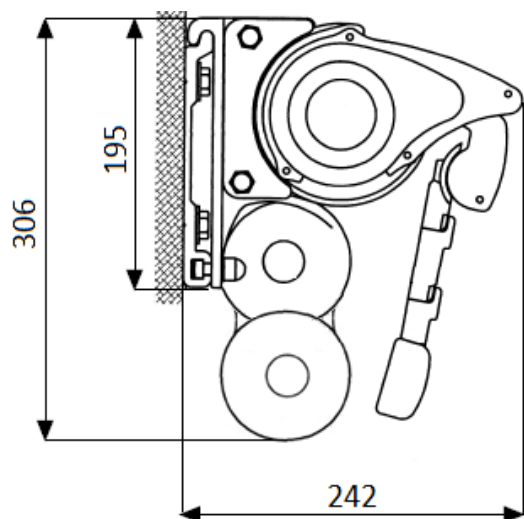
Vue de Coupe, Pose de Face:
