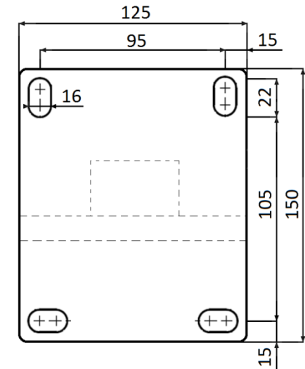
Détail Support/Platine Pose Plafond:
