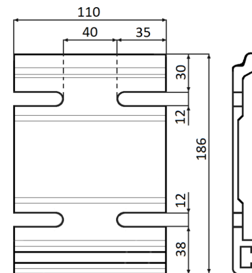
Détail Support/Platine Pose de Face:
