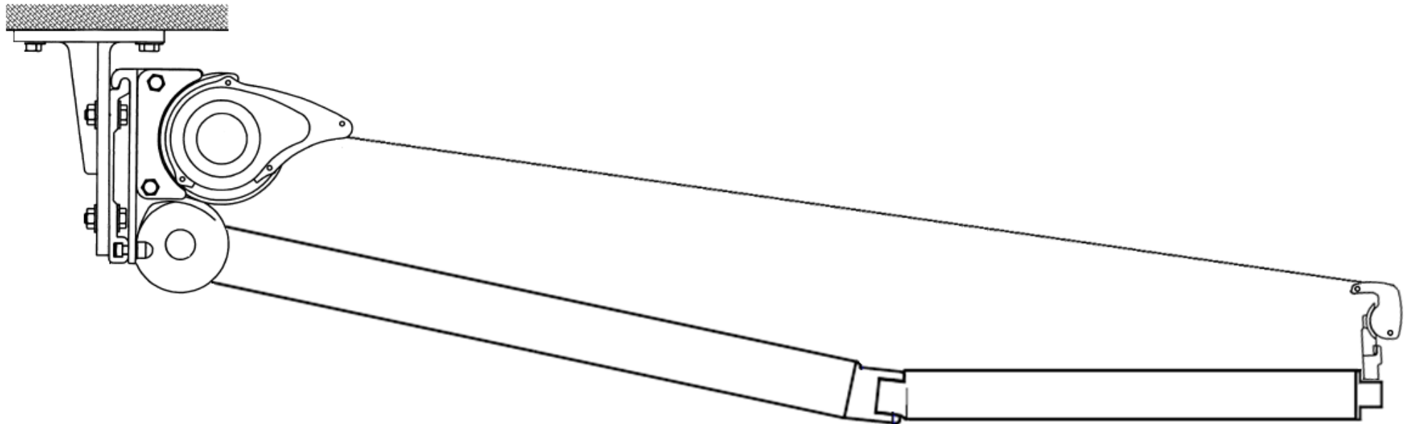
Vue de Côté, Pose Plafond, Store Ouvert:
