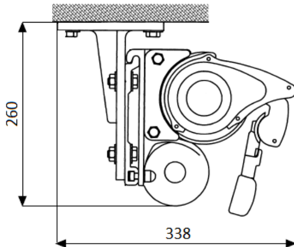
Vue de Côté, Pose Plafond, Store Fermé:
