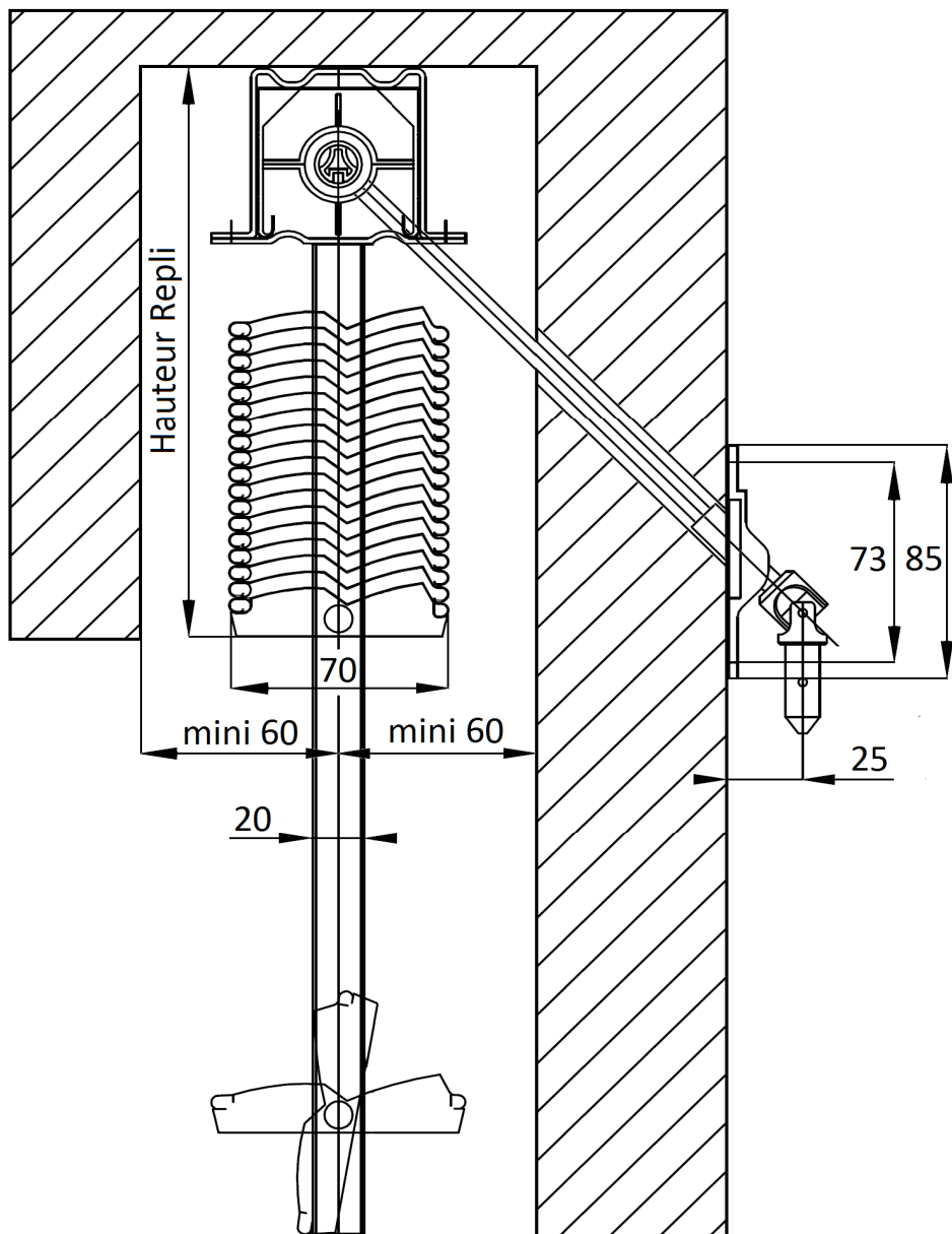
BSO 70 avec genouillère renvoi à 45° - Vue de coupe:
