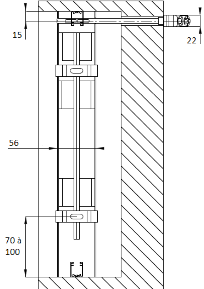
BSO 70 avec genouillère renvoi à 90° - Vue de dessus:
