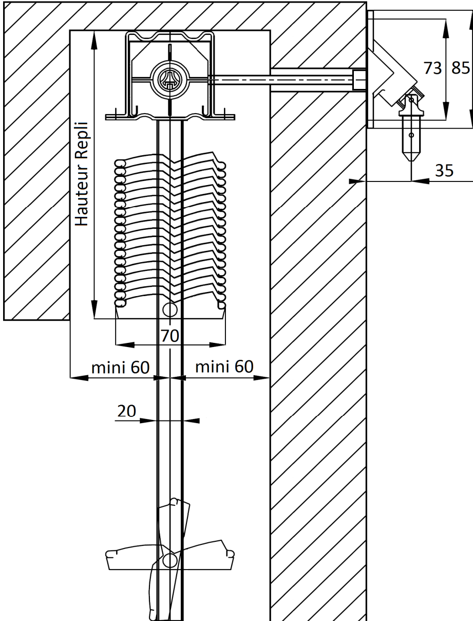
BSO 70 avec genouillère renvoi à 90° - Vue de coupe:
