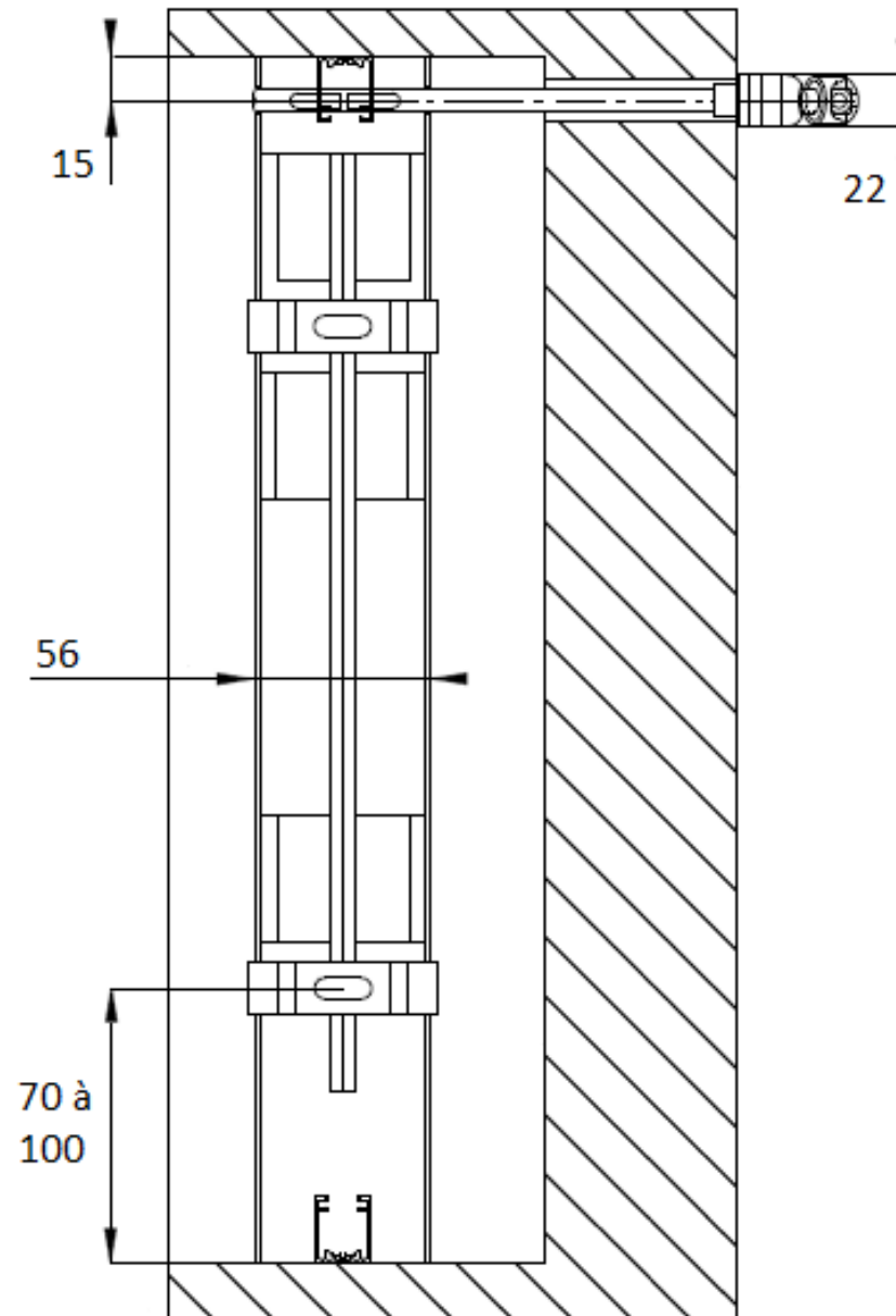
BSO 70 avec genouillère renvoi à 45° - Vue de dessus:
