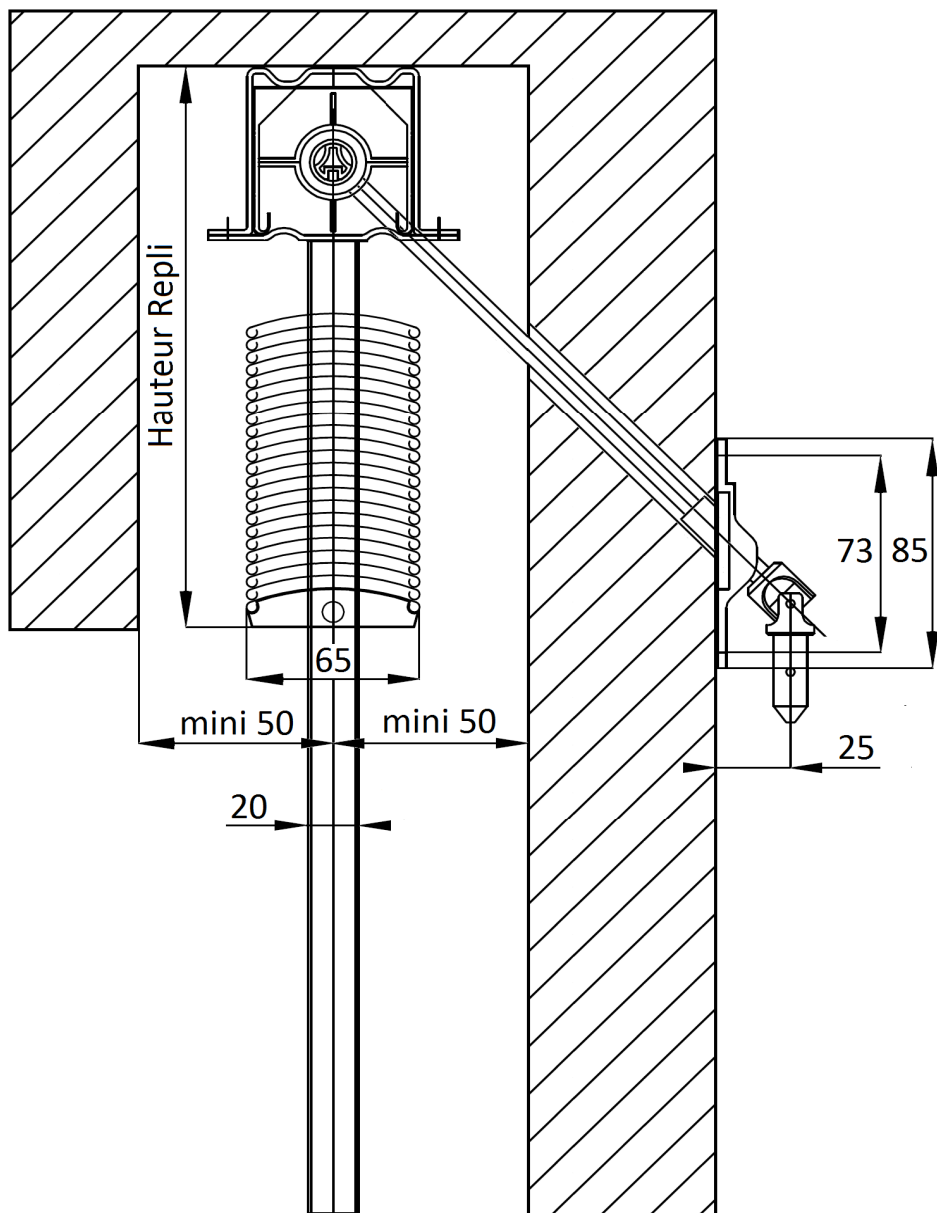
BSO 65 avec genouillère renvoi à 45° - Vue de coupe:
