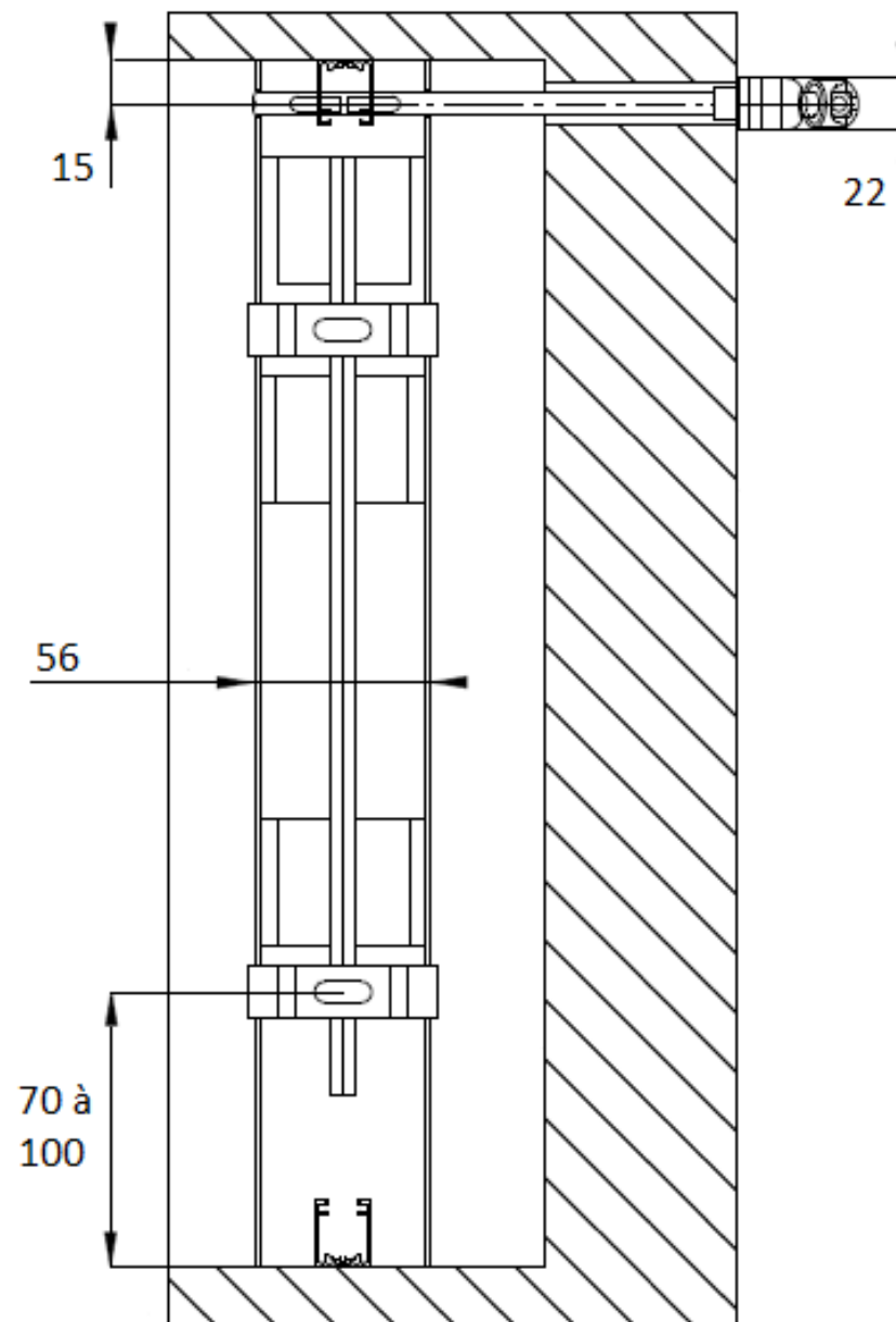
BSO 65 avec genouillère renvoi à 45° - Vue de dessus:
