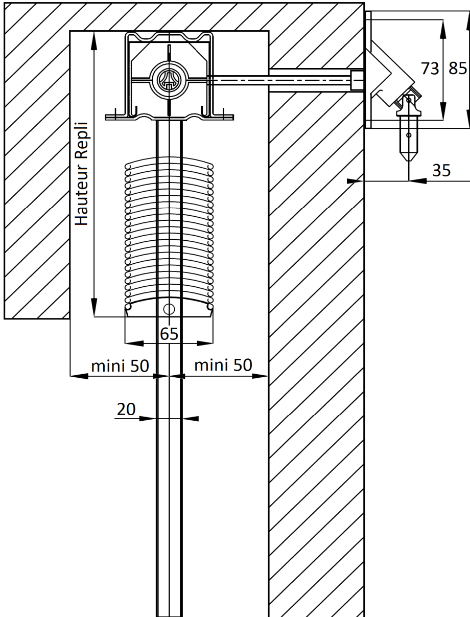
BSO 65 avec genouillère renvoi à 90° - Vue de coupe:
